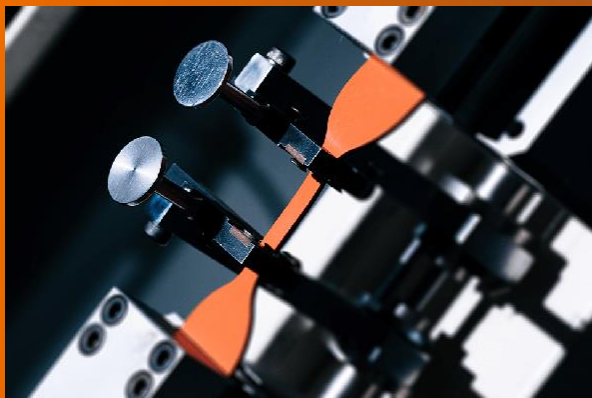
微電腦拉力測試機
