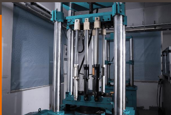
減震油封耐久試驗機
